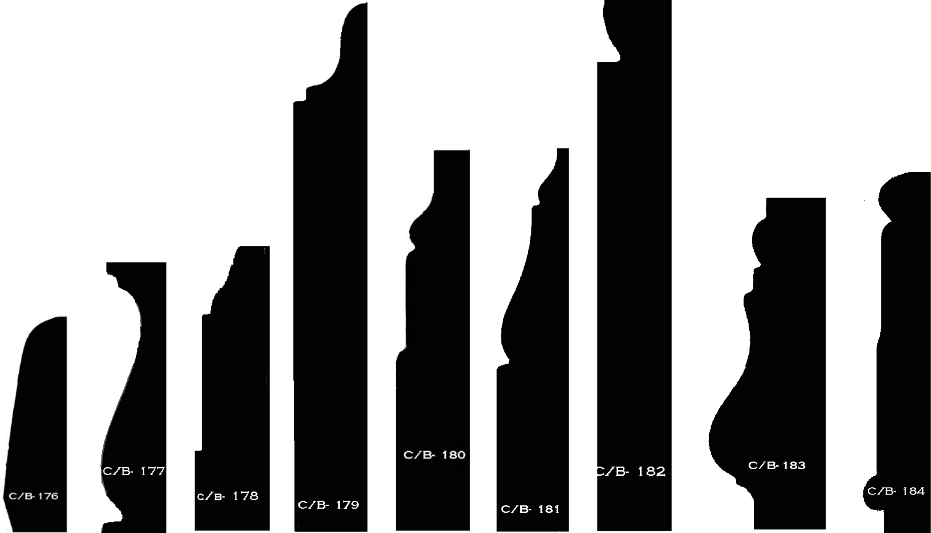
CB-176 CB-177 CB-178 CB-179 CB-180 CB-181 CB-182 CB-183 CB-184 2 1/4" 2 7/8" 3" 5 1/2" 4" 4" 6 3/4" 3 1/2" 3 3/4"
